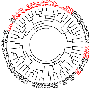
(d) K = 3
