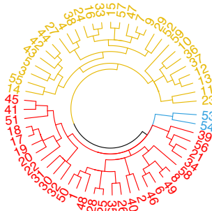
(d) K = 3
